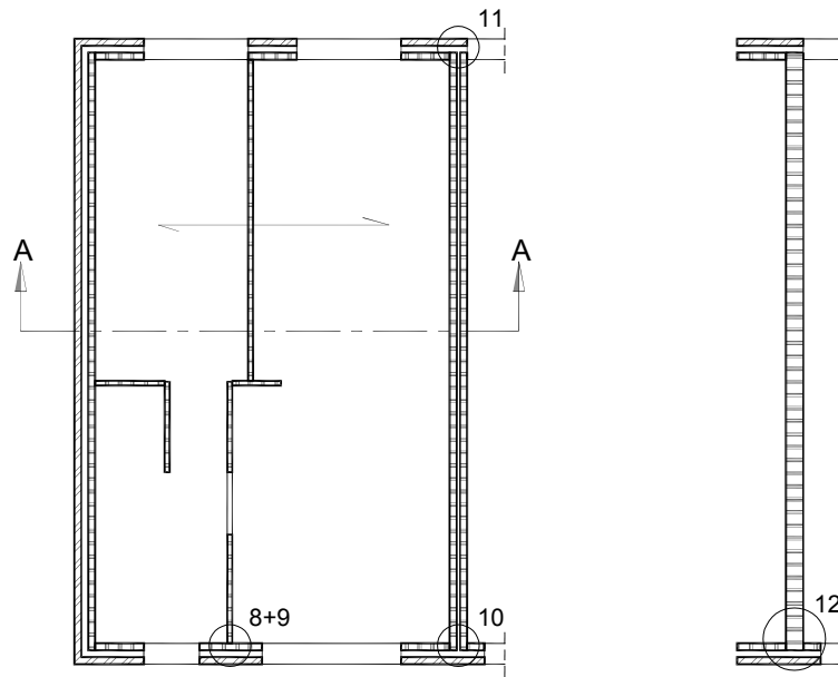
PLATTEGROND
