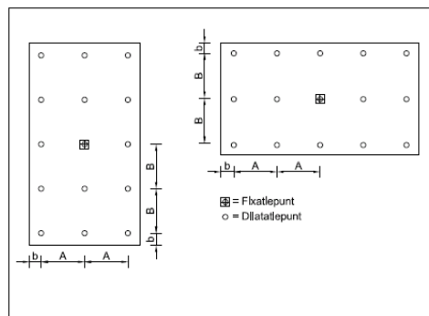
Figuur 4: 3-puntsbevestiging
