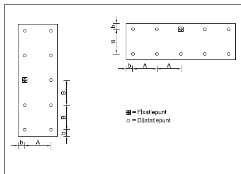
Figuur 3: 2-puntsbevestiging
