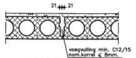
voegdetail 13
