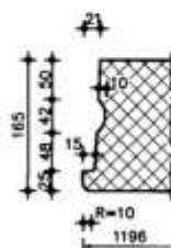
kelkvoegdetails
