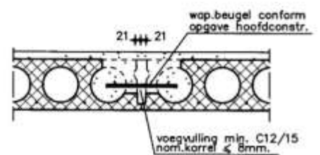
voegdetail 13A
