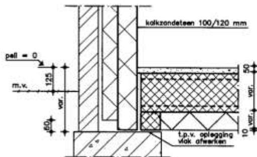
begingrond kalkzandsteendetail 7
