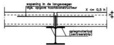
detail 12 – langsvoeg
