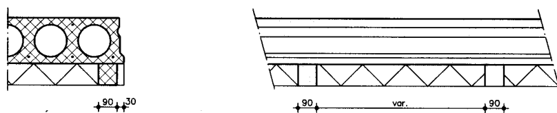
zijaanzicht t.p.v. oplegnokken
