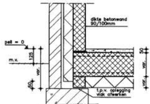
begingrond betondetail 2
