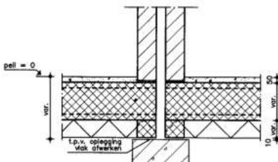
Indien wand woningscheidend zie tabel 6 begingrond detail 3A
