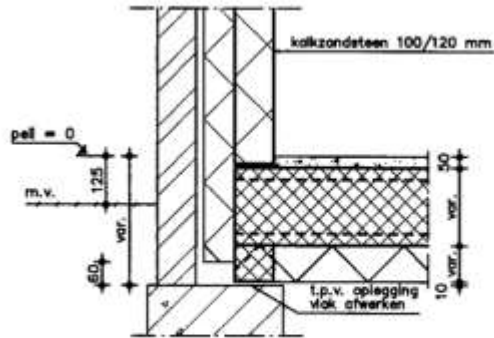
begingrond kalkzandsteendetail 2
