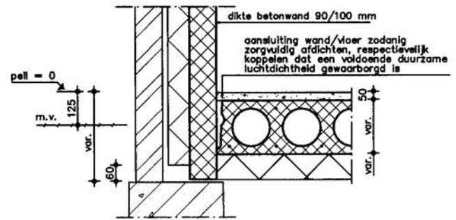
beganegrond betondetail 10
