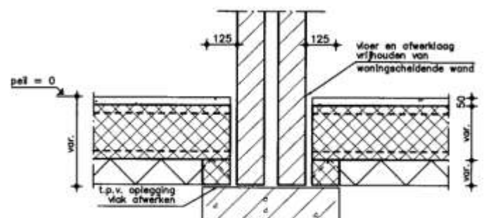
Indien wand woningscheidend zie tabel 6 begingrond detail 3B
