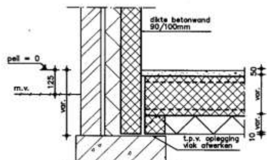
begingrond betondetail 7
