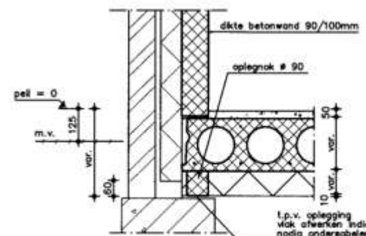
begangrond detail 6 tussensteunpunt
