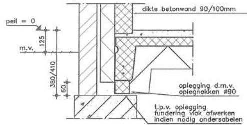
betondetail 6
