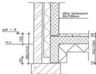
betondetail 1A
