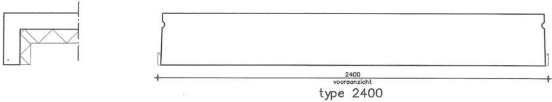
ongeisoleerd kopschot
