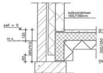
kalkzandsteendetail 1A
