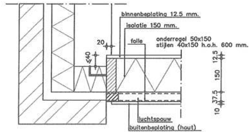
horizontale aansluiting vliesgevel Rc-gevel \geq 2,5 m 2 K/W
