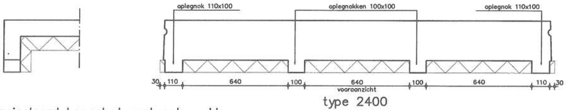
geisoleerd kopschot met oplegnokken
