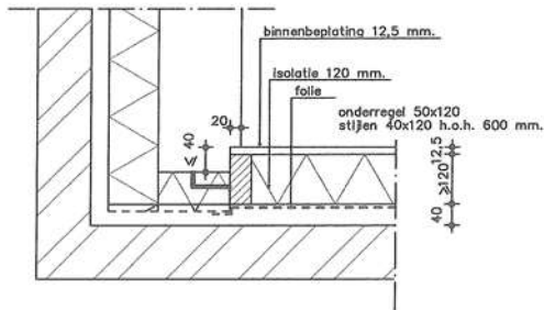
horizontale aansluiting houten binnenspouwblad Rc-gevel \geq 2,5 m 2 K/W
