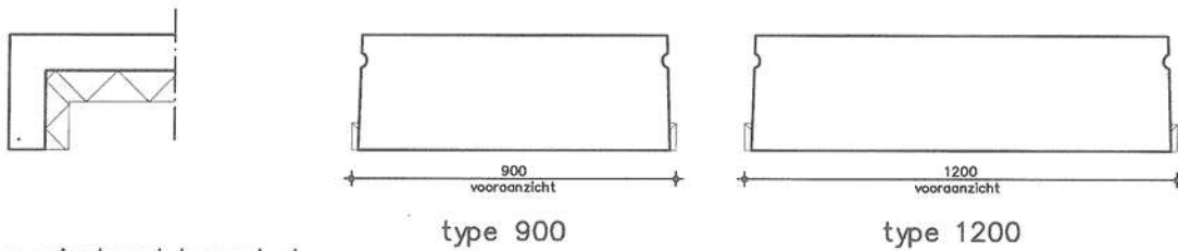
ongeisoleerd kopschot
