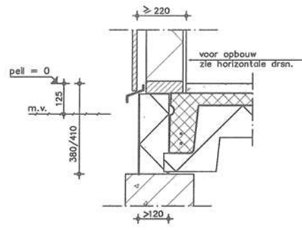
detail 6 – vliesgevel
